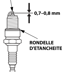
ELECTRODE LATÉRALE
