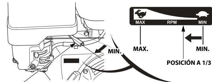
PALANCA DEL ACELERADOR
