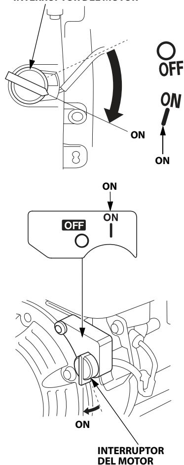
INTERRUPTOR DEL MOTOR
